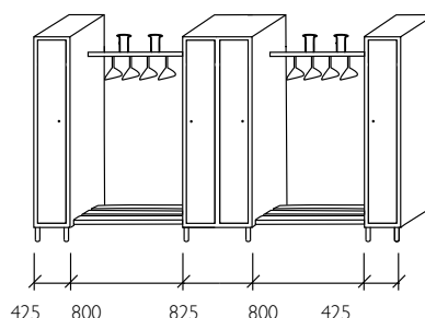
Aufstellungsbeispiel
