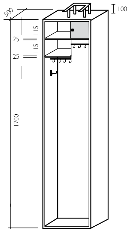
Serie 205
