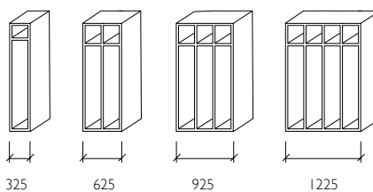
Serie 601
