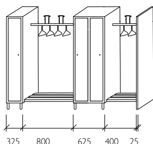
Serie 130 Aufstellungsbeispiel
