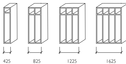
Serie 604
